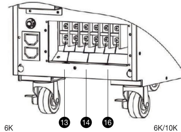
Diagrama 2: Terminal de entrada/salida
