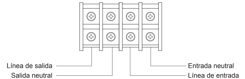
Diagrama de cableado del bloque terminal de 6 mil /10 mil
